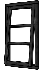
Uitzetraam enkel 04 Afmeting kozijn: 808x1430mm Afmeting raam: 674x1296mm
