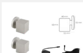
Down vierkant RVS Afmeting: 35x35x64mm Dimbaar
